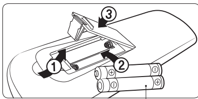
dvě baterie 1,5 V typu AAA
